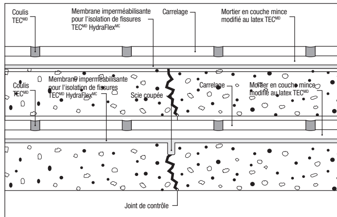
Fig. 1 : Traitement de fissures ou de joints de contrôle avec la membrane d'isolation étanche de fissures TEC HydraFlex
