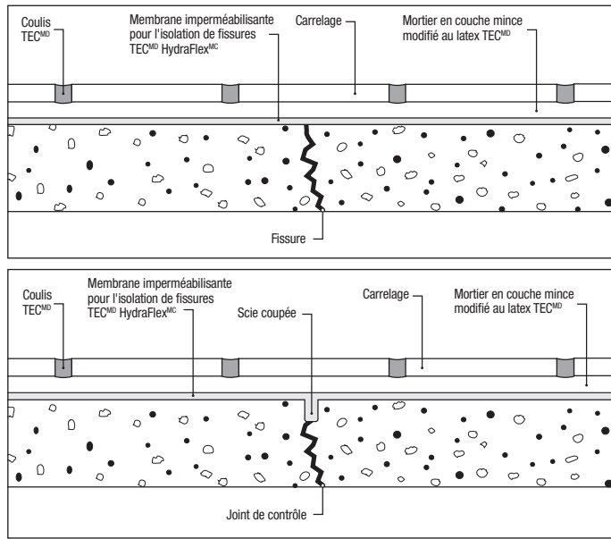
Fig. 1 : Traitement de fissures ou de joints de contrôle avec la membrane d'isolation étanche de fissures TEC MD HydraFlex MC
