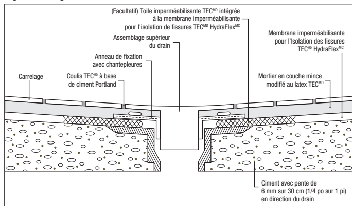
Fig. 2 : Configuration du drain
